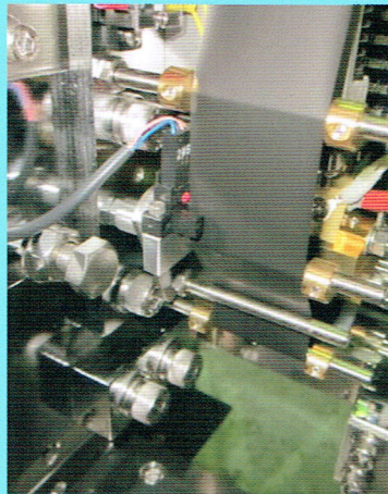
印字テープ切れセンサーの取り付け
