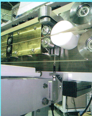
噛み込みセンサーの取り付け
