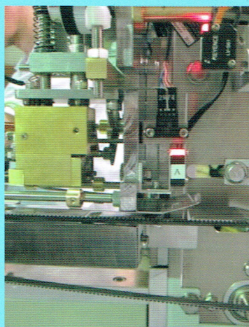
レーザーセンサーの取り付け
